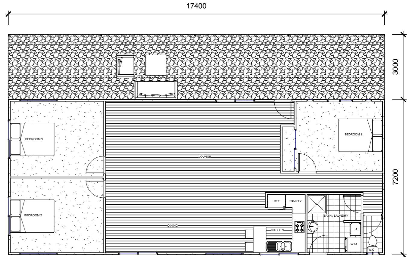
1 Floor Plan 1 : 100
